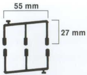
3-spårs rälsprofil
