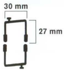
2-spårs rälsprofil
